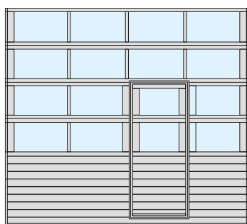
ВОРОТА С ПРОХОДНОЙ ДВЕРЬЮ И АЛЮМИНИЕВОЙ ПАНЕЛЬЮ СО СТЕКЛОПАКЕТОМ
