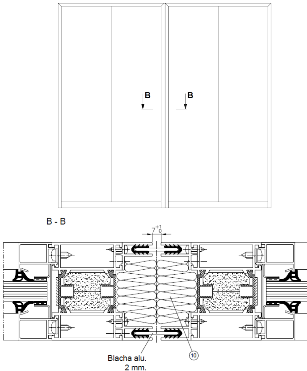
Rys.16. Połączenie dylatacyjne ścian słupowo-ryglowych i bezsłupkowych
