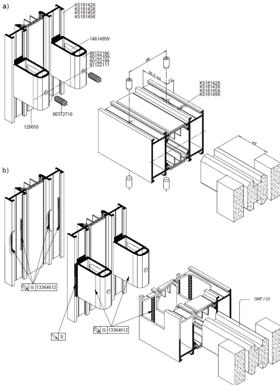
Rys.14. Połączenia typu „T” elementów konstrukcyjnych ścian : a) elementy łączące , b) uszczelnienie połączeń
