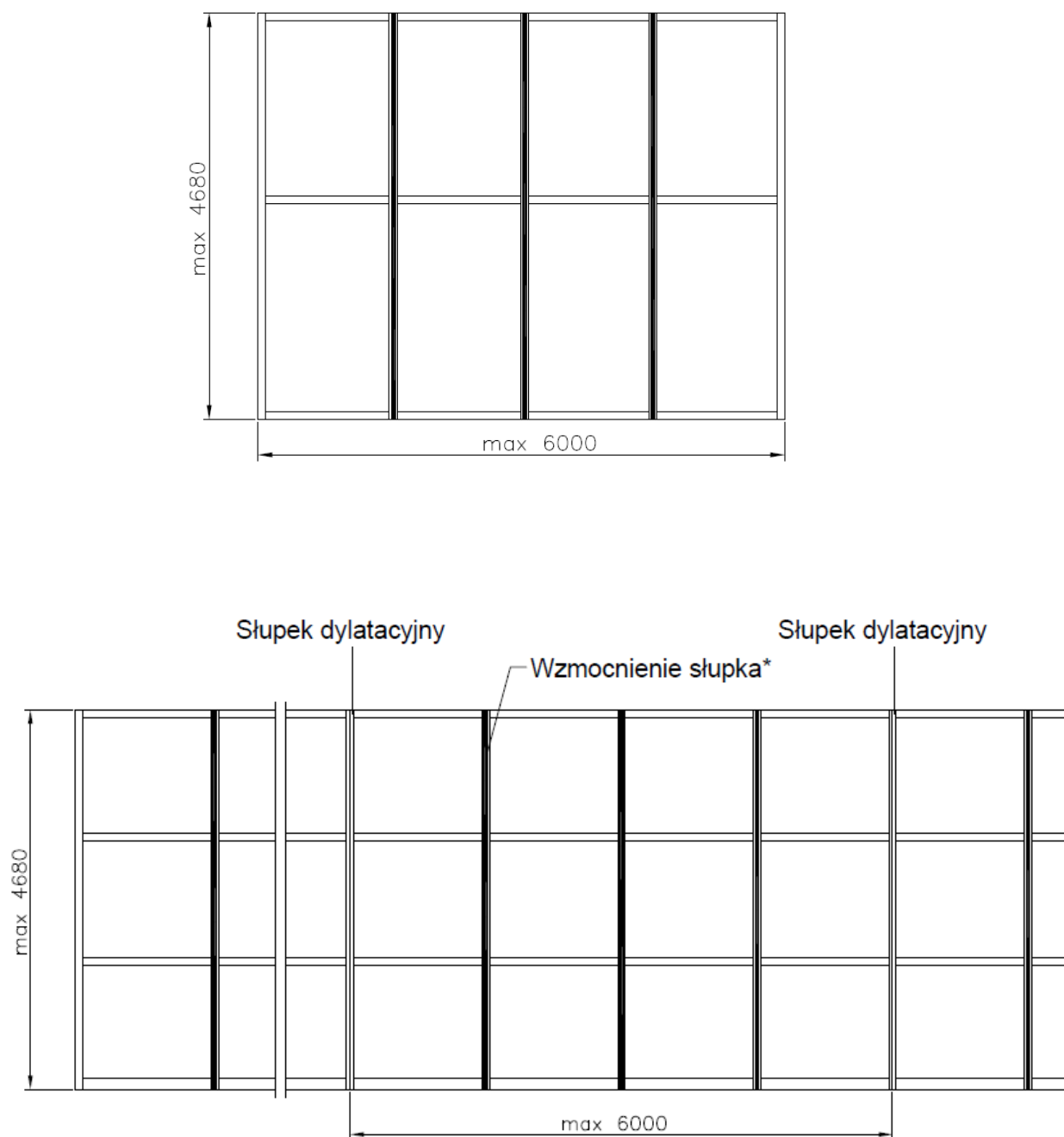
Rys.5. Maksymalne wymiary ścian słupowo-ryglowych MB-78EI w klasach EI30 i EI60 o słupkach wzmocnianych ( warunki wzmocnienia słupków podano w tablicy 3
