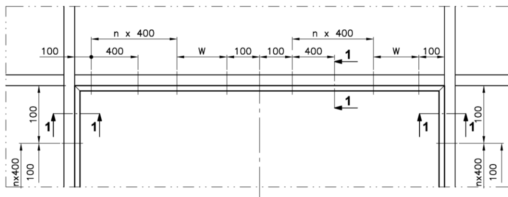
Rys. 21. Montaż listwy przymykowej K518139X
