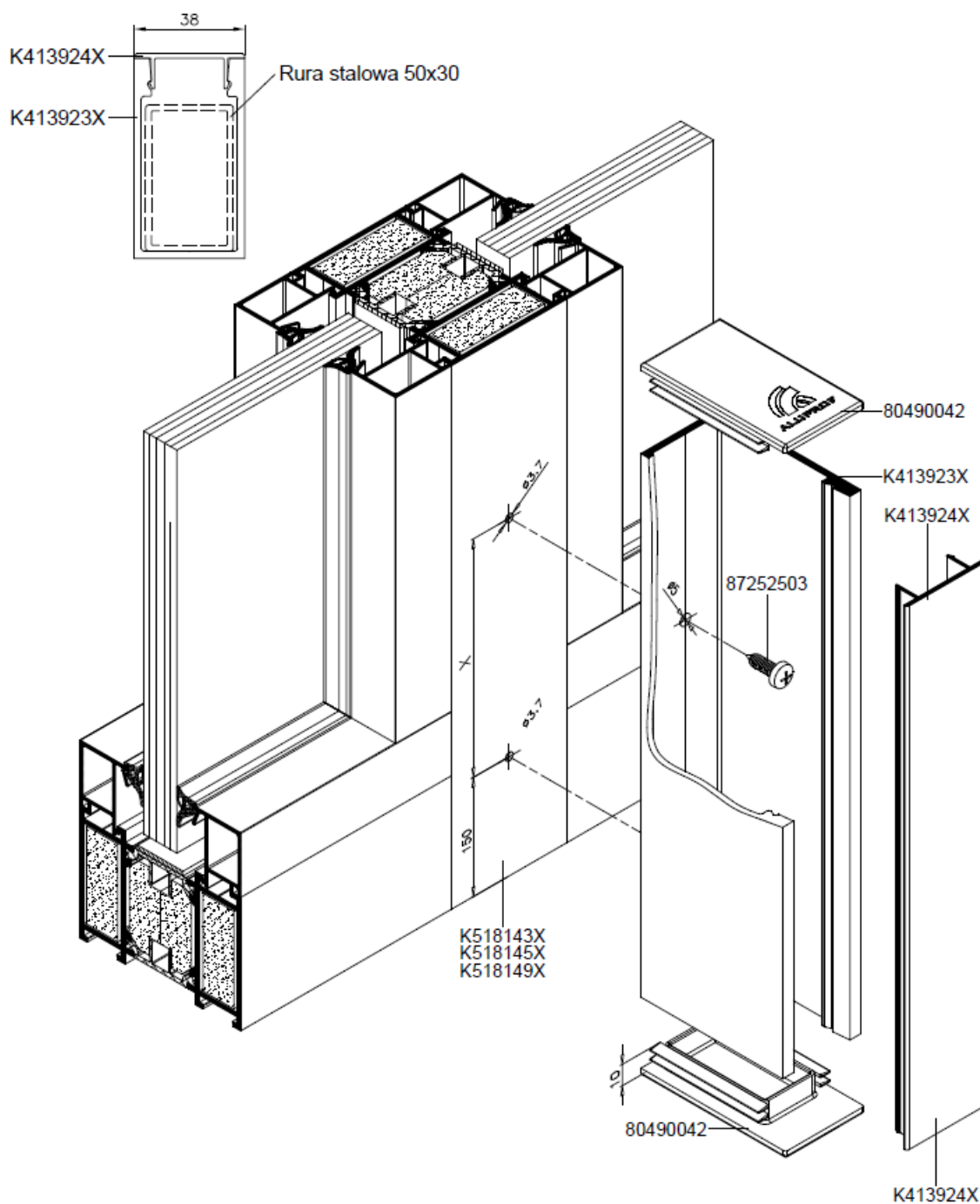
Rys.20. Montaż wzmocnienia słupka wysokiej ściany ogniodpornej .
