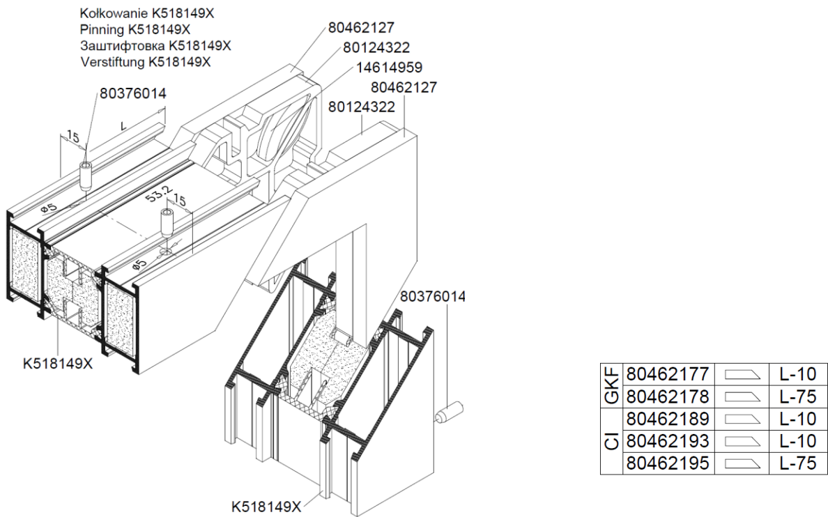
Rys.12. Elementy połączenia typu "L" naroży ram ściennych metodą kolkowania-rama z kształtownika K518149X
