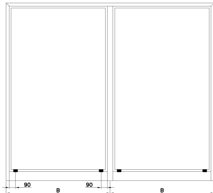
Rys.33. Rozmieszczenie podkładek podszybowych w ścianach bezslupkowych i slupowo-ryglowych
