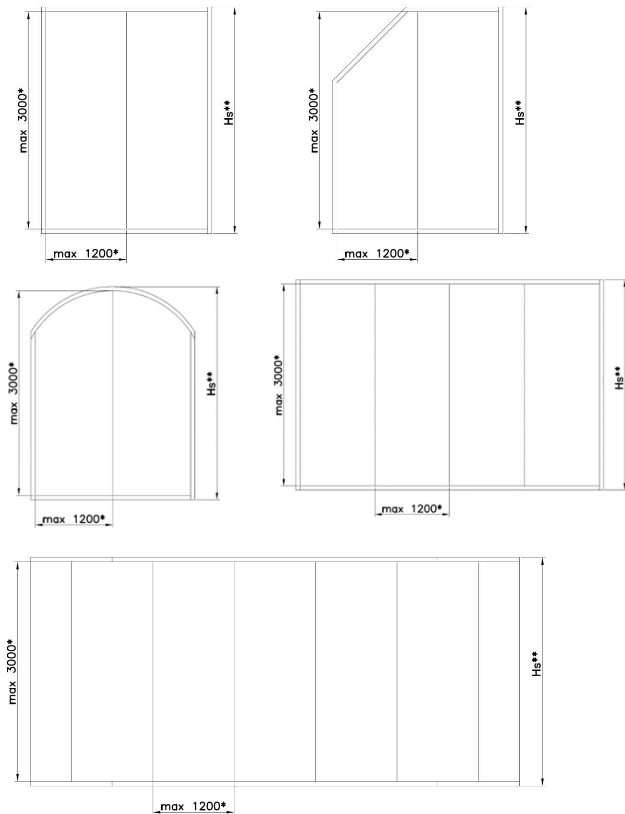
1 Rys. 6. Maksymalne wymiary ścian bezsłupkowych
