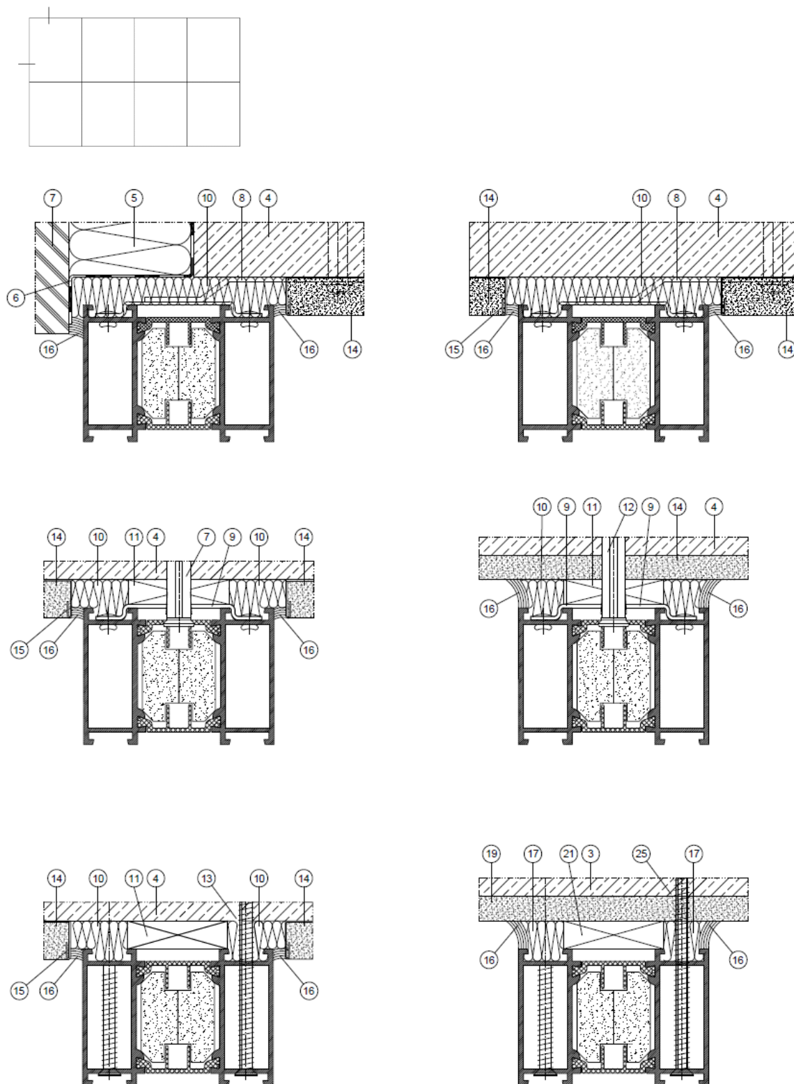
Rys.17. Przykłady uszczelnienia połączenia ram ścian zewnętrznych i wewnętrznych MB-78EI z konstrukcją budynku
