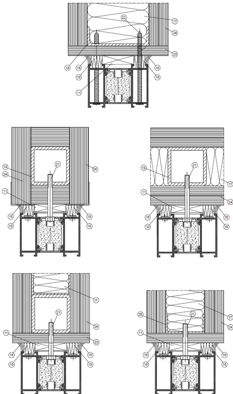
Rys.19 Warianty uszczelnienia połączenia ościeżnic i ram montowanych w ścianach podatnych, np. z okładziną z płyt kartonowo -gipsowych
