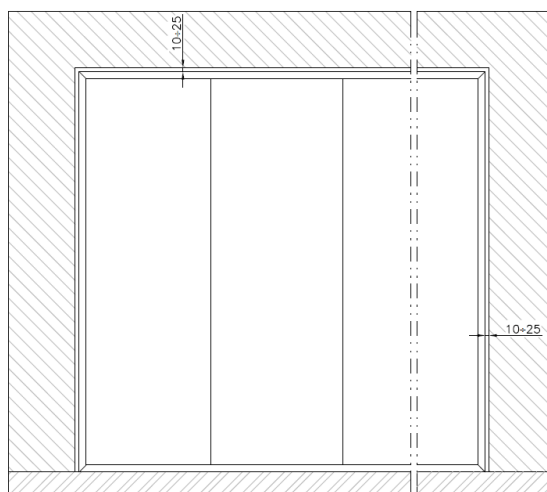
Rys.1. Standardowe luzy między wymiarami otworu budowlanego a ramą obwodową ściany przeciwpożarowej : a) ściana słupowo-ryglowa , b) ściana bezsłupkowa
